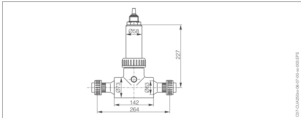
Chambre de passage FlowFit W CUA 250
