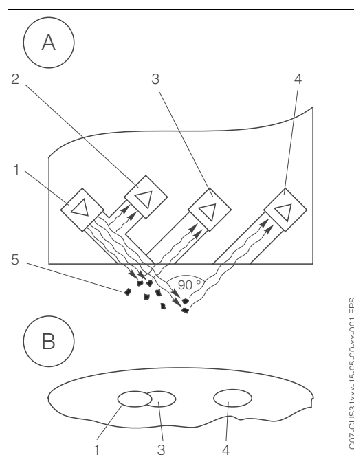
Mesure de la turbidité selon ISO 7027 / EN 27027
