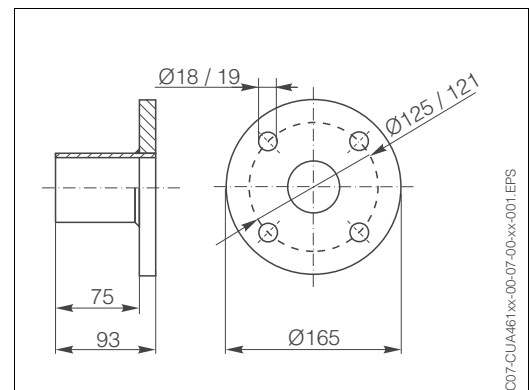
Manchon à souder pour CUA 461 ou CUA 120
