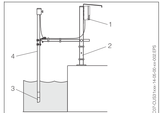
Ensemble de mesure avec sonde à immersion
