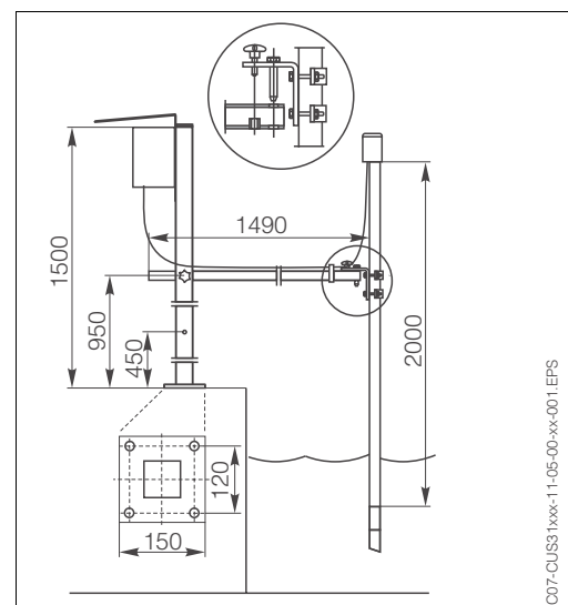
Support de sonde CYH 101 avec sonde CYA 611
