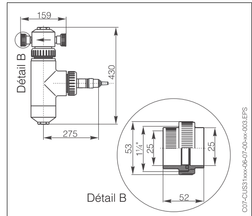
Chambre de passage S (avec dégazeur)
