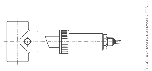
Orientation face à l'écoulement du produit
