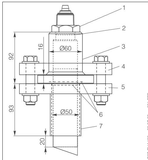
Adaptateur CUA 120-B avec raccord à souder DN 50 / ANSI 2" avec bride tournante
