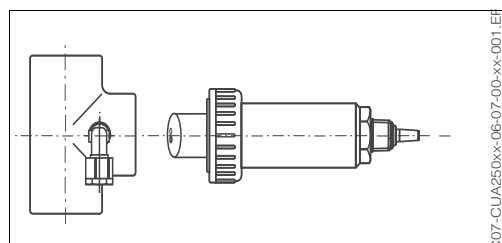
Orientation parallèle du capteur
