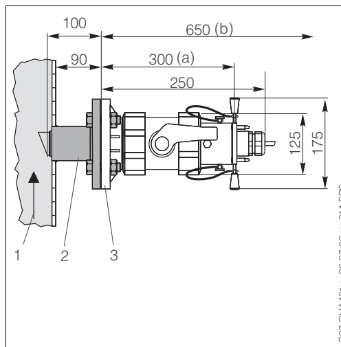
Sonde rétractable CUA 461
