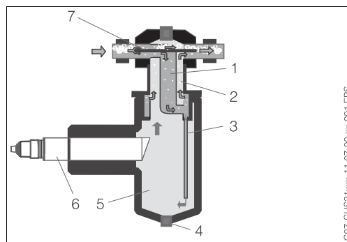
Chambre de passage S avec dégazeur intégré (sonde S)
