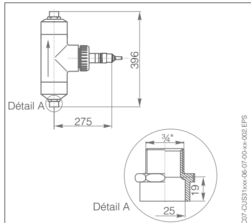
Chambre de passage E (sans dégazeur)
