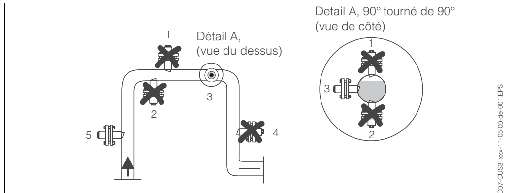
Positions de montage du CUS 31 avec adaptateur CUA 120-A/B ou avec sonde rétractable CUA 461
