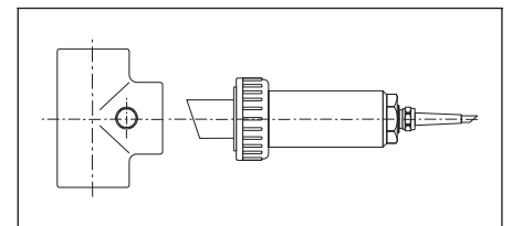
Installation contraire au sens d'écoulement du fluide
